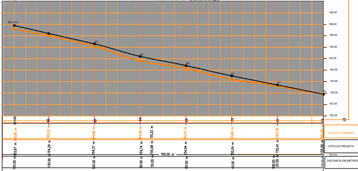
PERFIL DA RUA CACILDA ALVES GUIMARÃES
